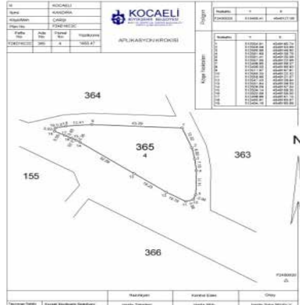
Aplikasyon Krokisi Örneği
